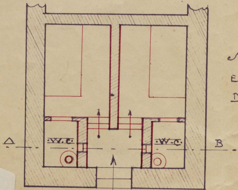
PLANTA.
